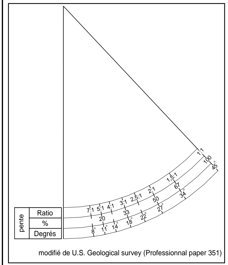
Figure 3 : Illustrations des diverses façons d'exprimer une inclinaison (A : en degré, en pourcentage et en proportion, B : correspondance entre les trois systèmes de mesure)
